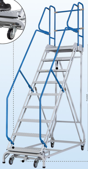
ML-2100B(9단) 790×1901×3039
